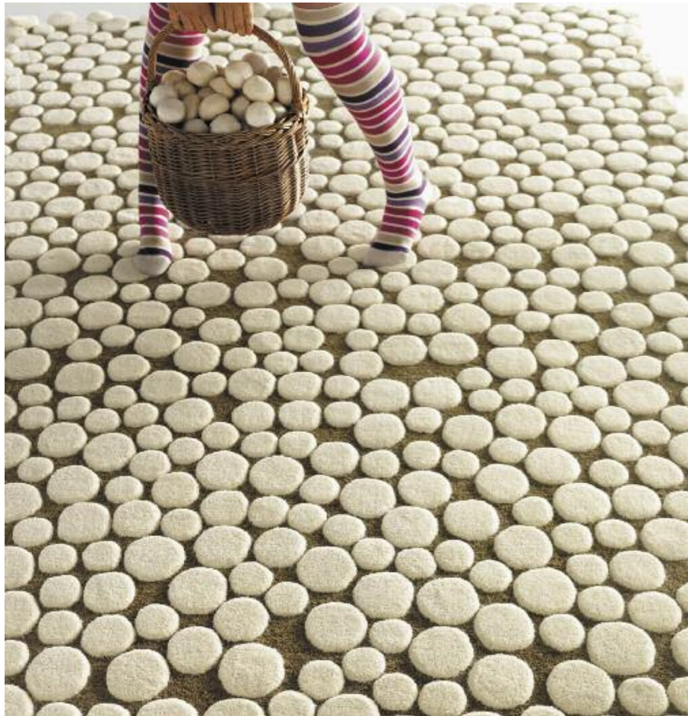
GAN
